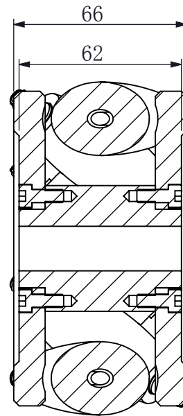
剖面 A-A
