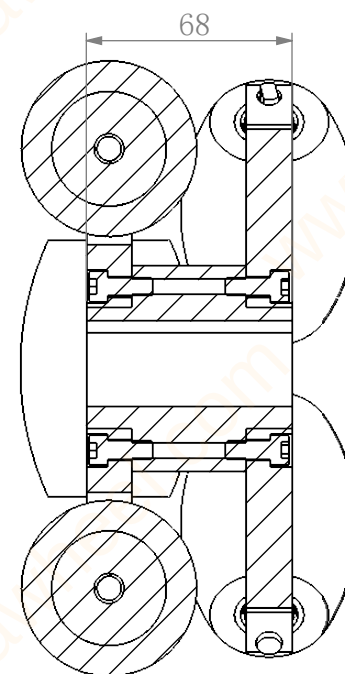
剖面 B-B 比例 1 : 2.5
