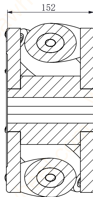
剖面 A-A 比例 1 : 4
