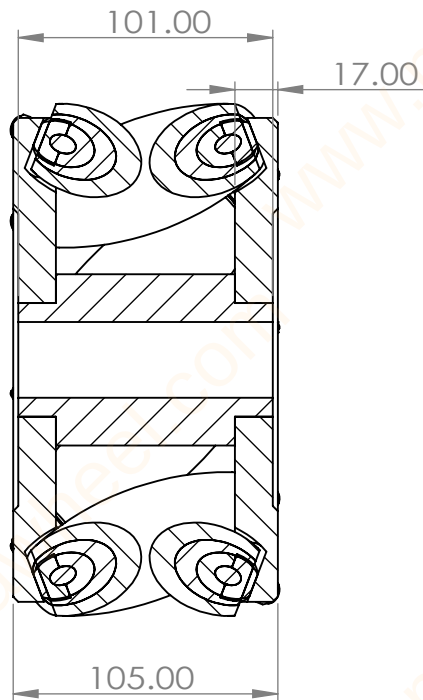
剖面 B-B 比例 1 : 3
